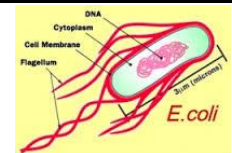
E. Coli
