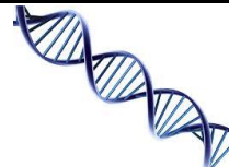
DNA streng
